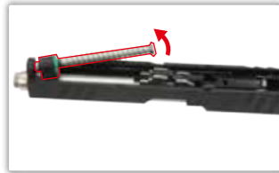
Retirer le guide ressort.
