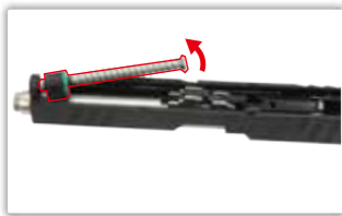
向前推擠覆進程後向上移出。
