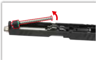
Retire la guía del muelle recuperador y el muelle recuperador.
