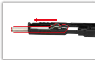
往前移動外管。
