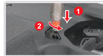
Utilisez un tournevis à tête plate, et tournez à 90 degrés dans le sens antihoraire.
